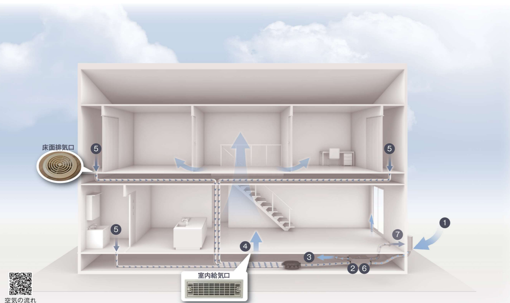
空気の流れ
